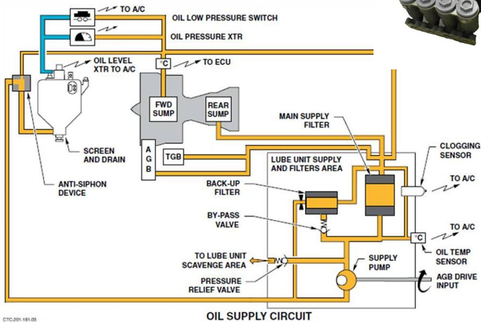
Lub Unit
